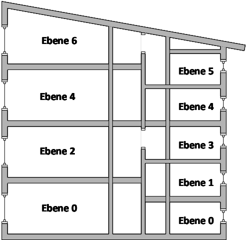
PRINZIPDURCHSCHNITT DURCH DAS GEBÄUDE
