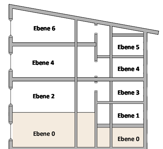
PRINZIP DURCHSCHNITT DURCH DAS GEBÄUDE
