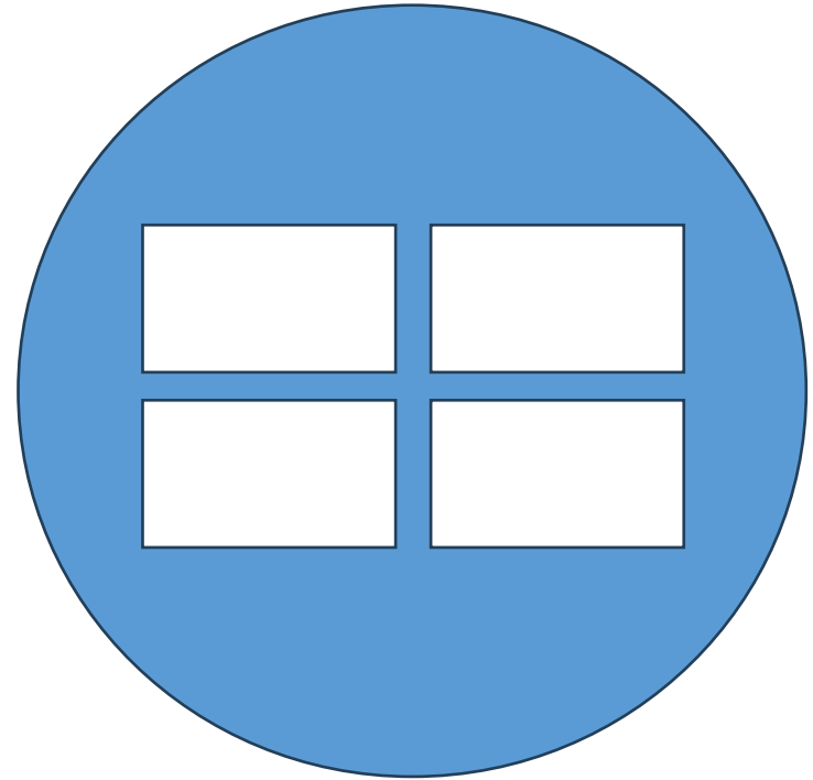
Abbildung 2: Vier Rechtecke im Kreis (eigene Darstellung)
