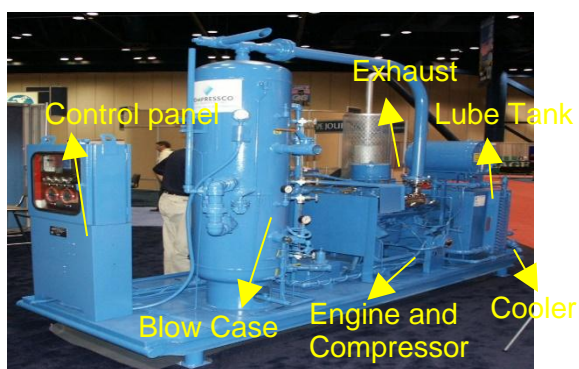
Figure 3. Mini Compressor Package
